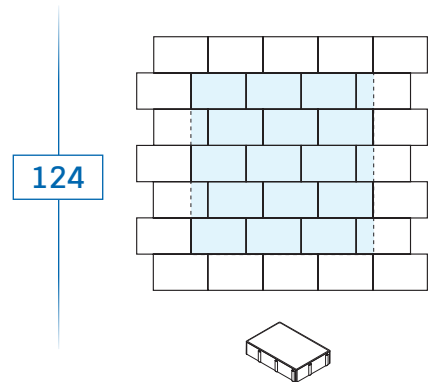
30 x 20 x 8 - environ 16,5 pces/m 2
