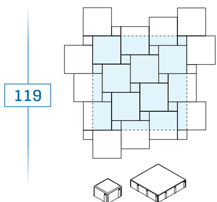
10 x 10 x 8 - environ 10 pces/m 2 30 x 30 x 8 - environ 10 pces/m 2
