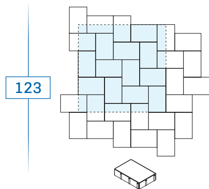
30 x 20 x 8 - environ 16,5 pces/m 2
