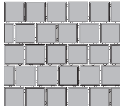
20 x 20 x 8 cm - environ 25 pièces/m 2
