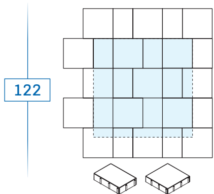
30 x 20 x 8 - environ 7 pces/m 2 30 x 30 x 8 - environ 7 pces/m 2
