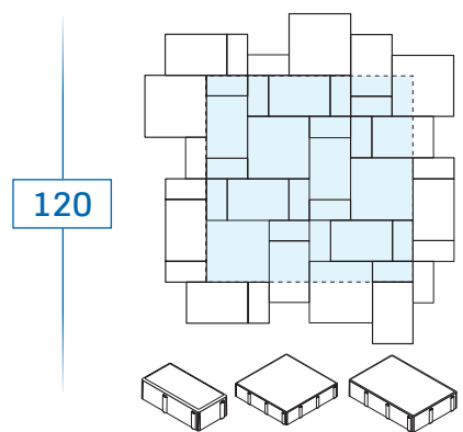
10 x 20 x 8 - environ 14 pces/m 2 30 x 20 x 8 - environ 6,5 pces/m 2 30 x 30 x 8 - environ 3,5 pces/m 2
