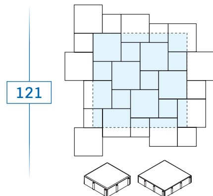
20 x 20 x 8 - environ 7,5 pces/m 2 30 x 30 x 8 - environ 8 pces/m 2
