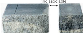
Élément de base 34 x 25 cm Poids / pce : 29,4 kg Élément de base 16 x 25 cm Poids / pce : 14,6 kg
